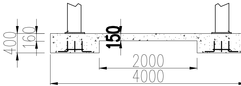
MẶT CẮT B-B
