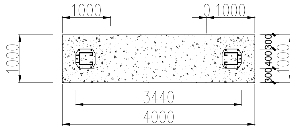
CHI TIẾT HỐ MÓNG CẦU NÂNG 2 TRỤ
