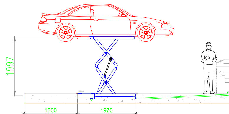
MẶT BẰNG LẮP THIẾT BỊ CẦU NÂNG CẮT KÉO HL-35F
