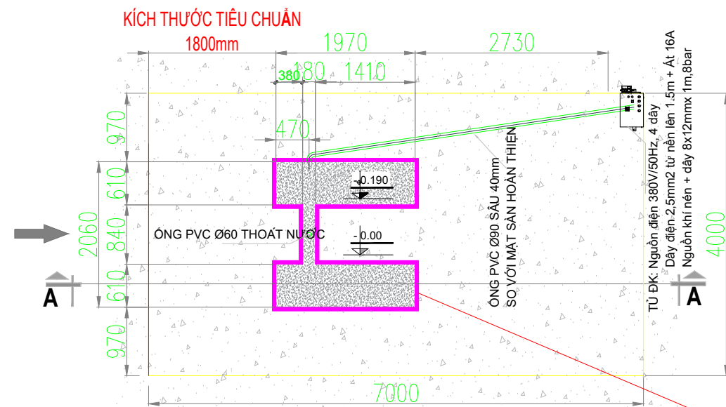
MẶT BẰNG HỒ MÓNG CẦU NÂNG CẮT KÉO HL-35F
