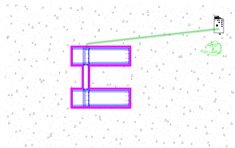
MẶT BẰNG LẮP THIẾT BỊ CẦU NÂNG CẮT KÉO HL-35F
