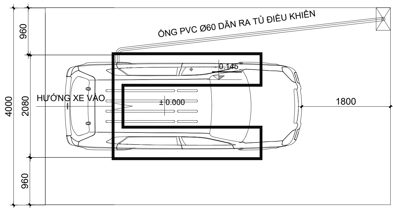
LAYOUT CẦU NÂNG CẮT KÉO 4.0m x 7.0m TỈ LỆ 1/50
